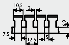
Bauhöhe 25
