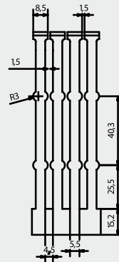
Bauhöhe 120
