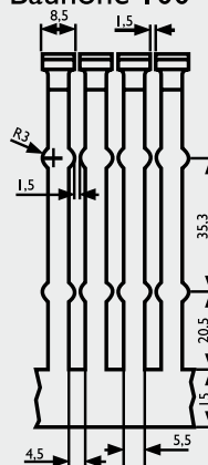
Bauhöhe 100
