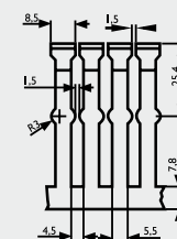
Bauhöhe 60
