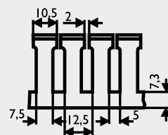
Bauhöhe 37,5
