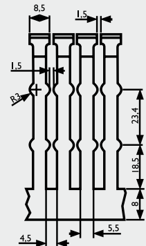
Bauhöhe 80
